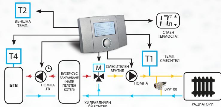
Постоянна температура в БГВ и управление на смесителя според външната температура
