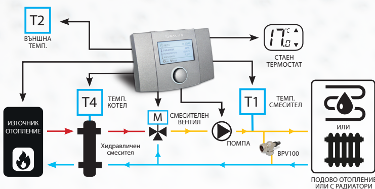
Регулиране на отоплителната система по външна темп.
